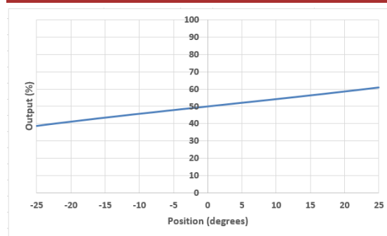
Linear Range
